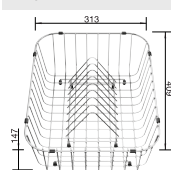
Multifunkčný kôš na riad s odnímateľným stojanom na tanier
