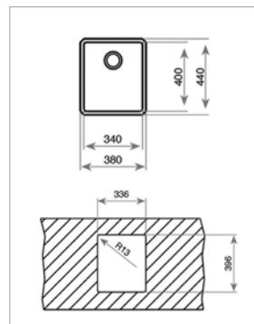
BE LINEA RS15 34.40
