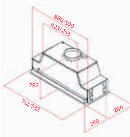
GFL 77760 - GFL 57760 GFL 57651
